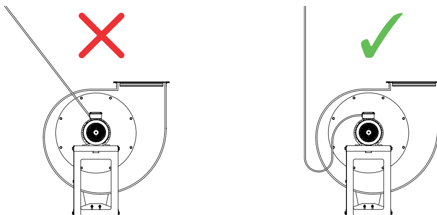
Рисунок 6.1 – Схема расположения силового кабеля
